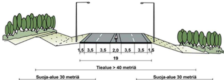
Kuva 1-5. Valtatien poikkileikkaus välillä Korpilahti-Muurame.
