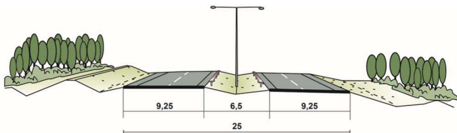
Kuva 1-6. Valtatien poikkileikkaus välillä Muurame-Keljonkangas.
