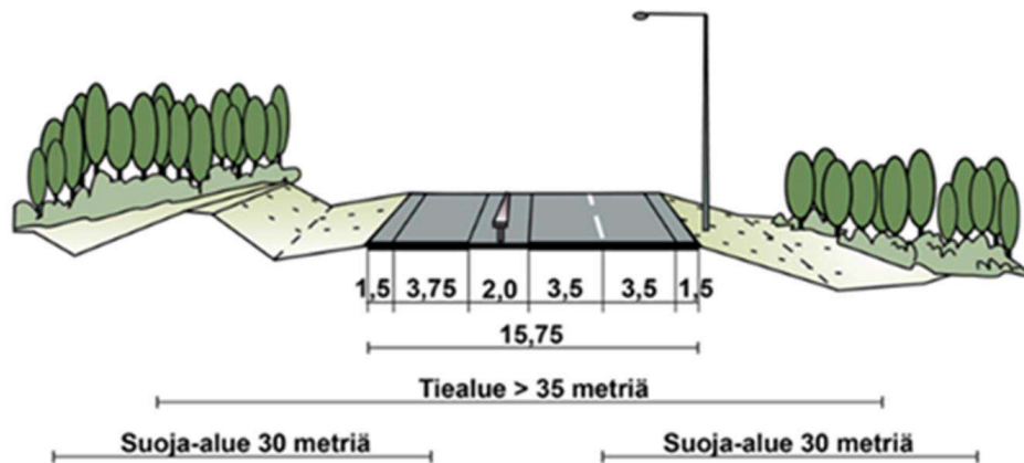
Kuva 1-4. Valtatien poikkileikkaus välillä Painaa-Korpilahti.
